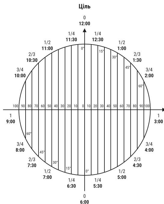
Рис. 1. Сітка поправкових коефіцієнтів урахування вітрового чинника
